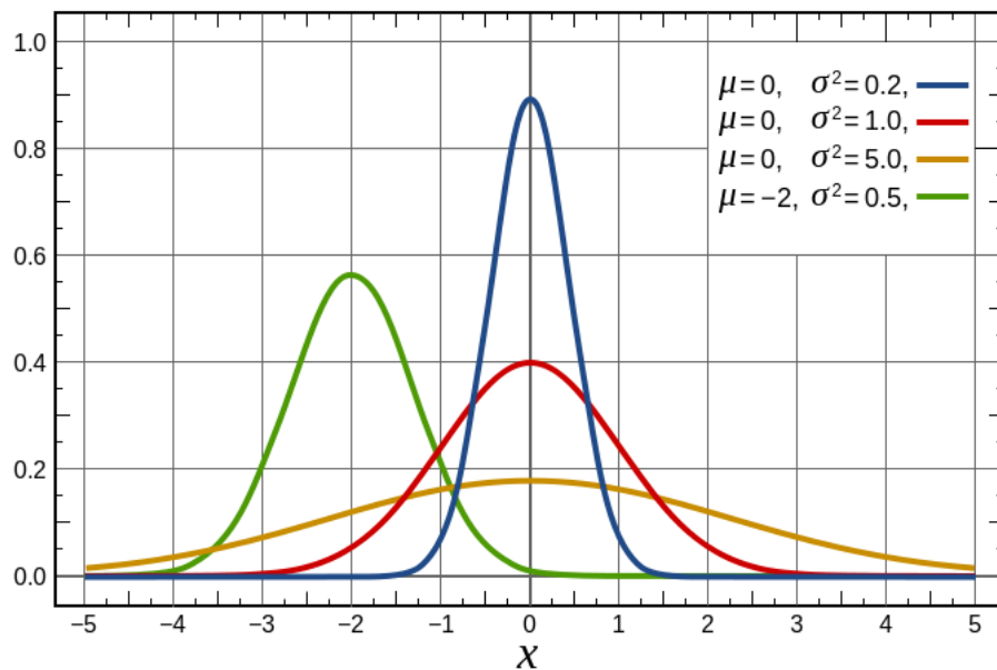
Σχήμα 5: Κανονική Κατανομή
