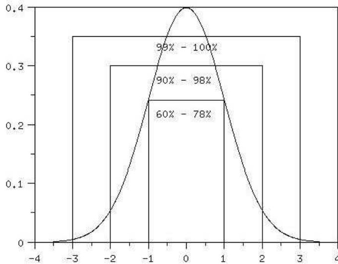
Σχήμα 4: Εμπειρικός Κανόνας
